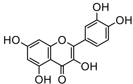
ケルセチン
