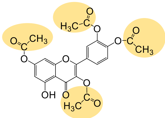
4Ac-Q
